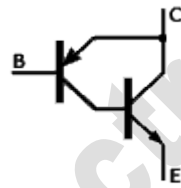
Transistor Sziklai
